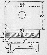
FANG CLIP E
