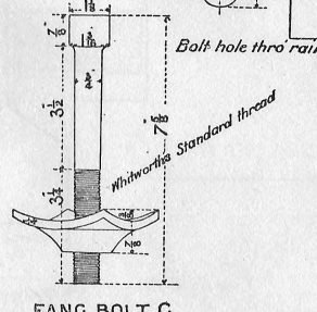
FANG BOLT C
