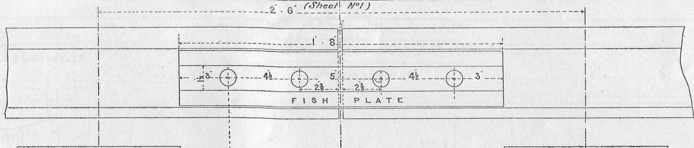
ELEVATION
