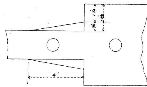
— Fig 6 — — SECTION C.C. —
