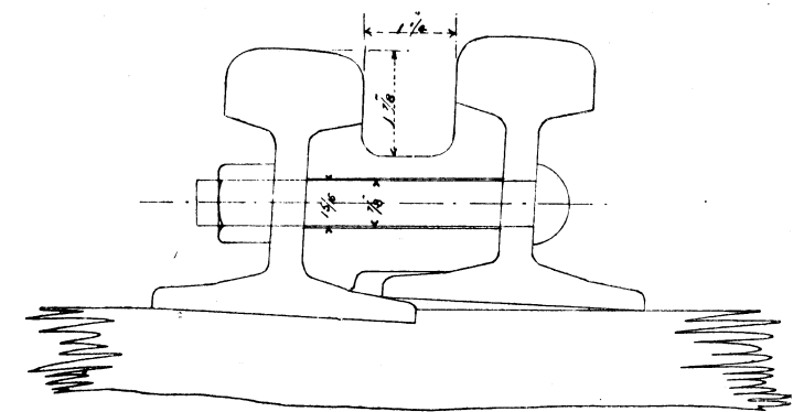
— Fig 7 — — SECTION B.B. —
