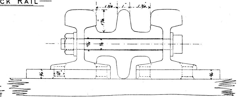
— Fig 4 — — SECTION E.E. —
