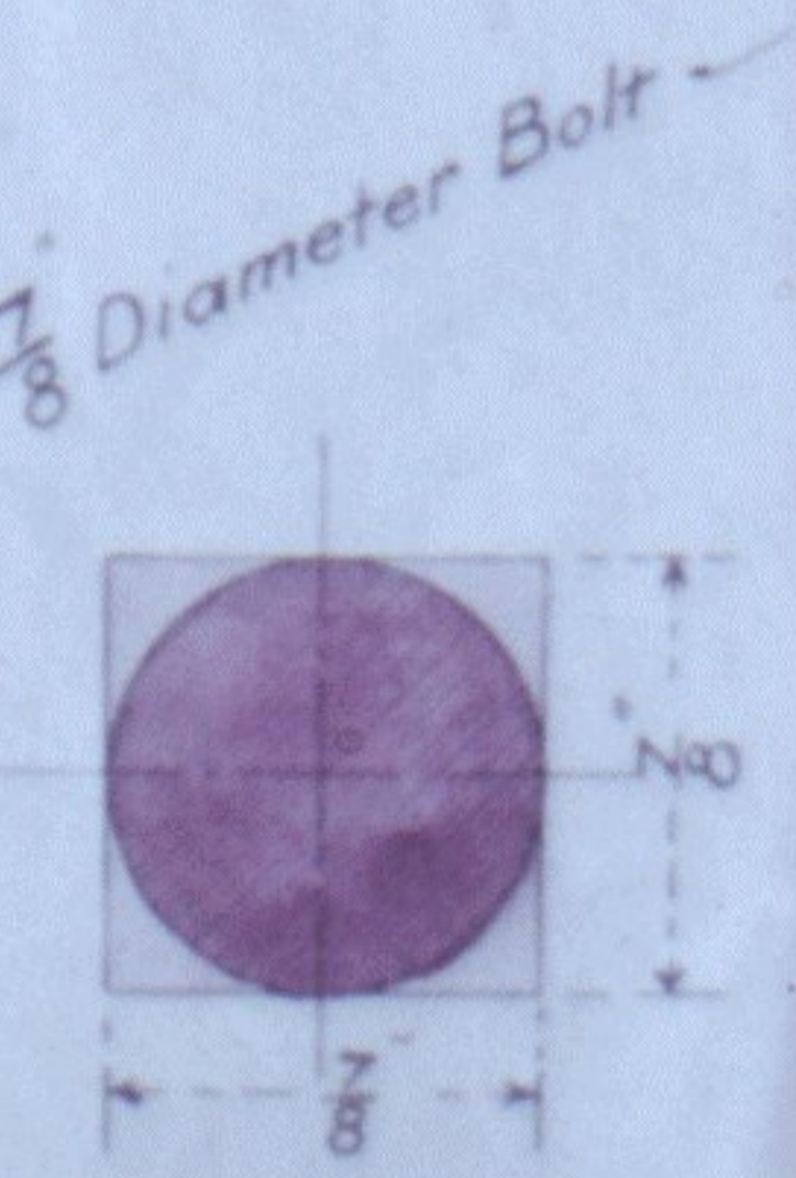
SECTION THRU A. A.
