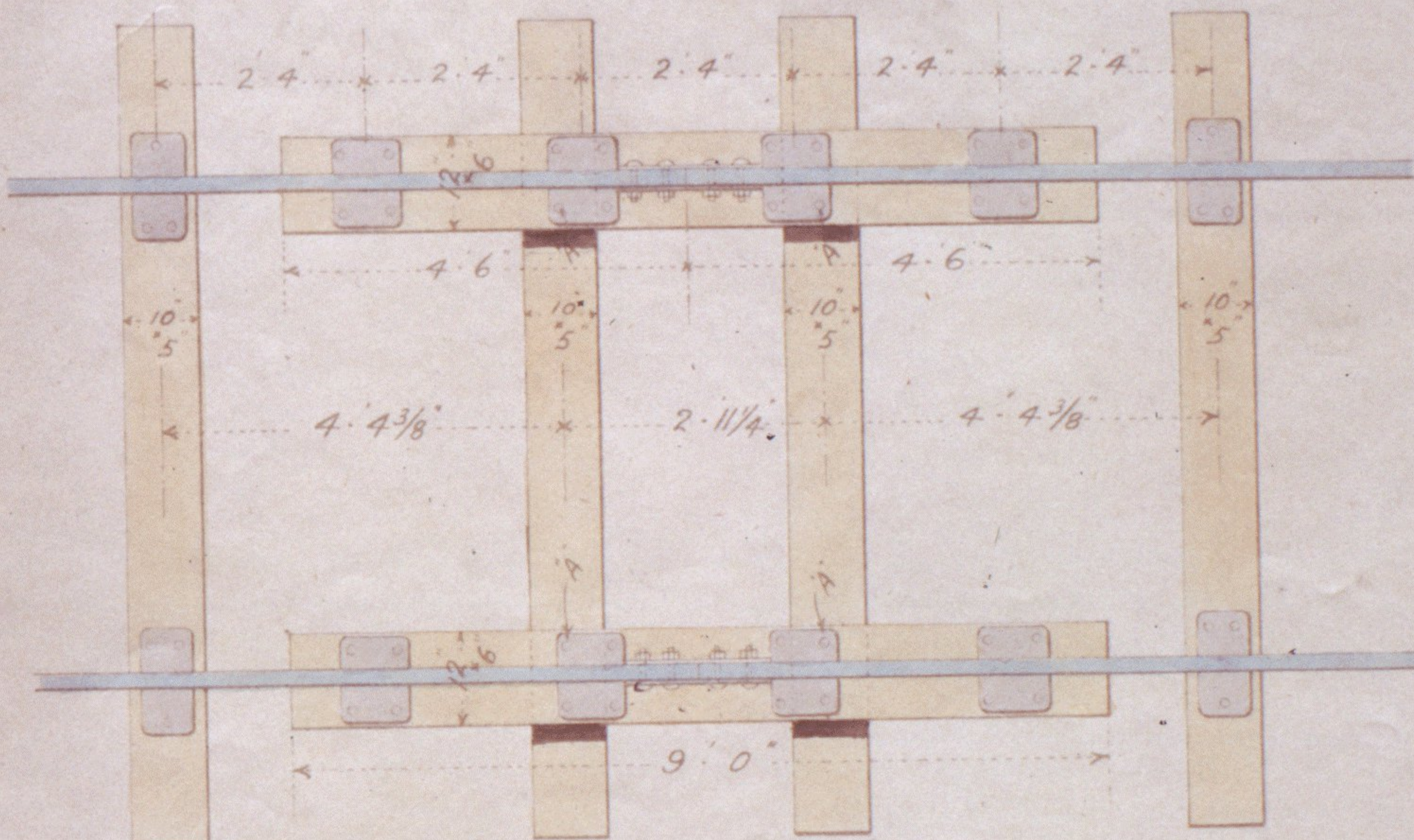
PLAN.
